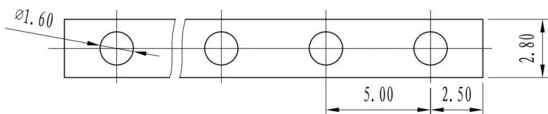
P.C.B. LAYOUT
